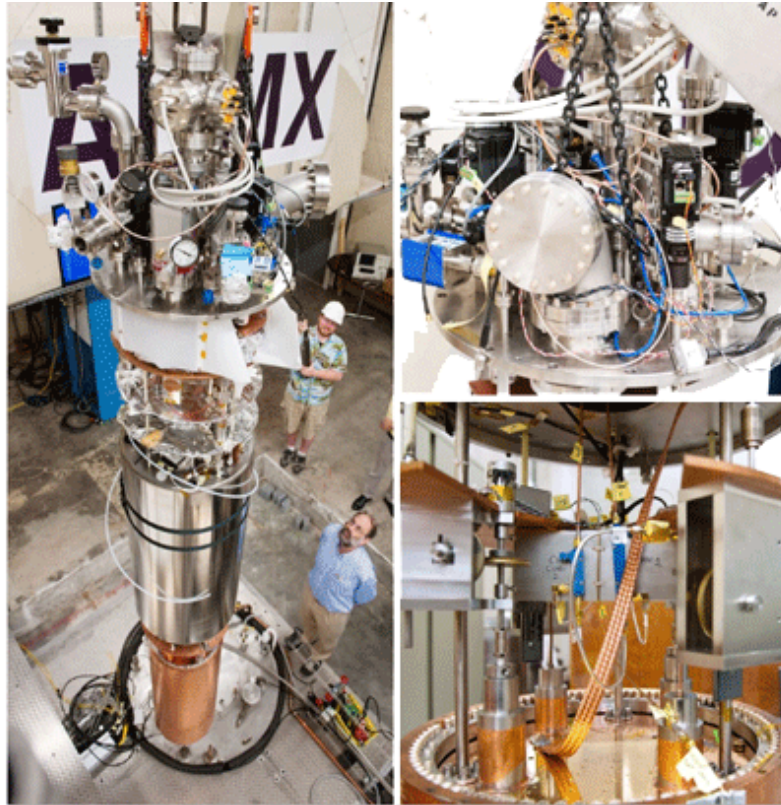
Detector de posibles axiones ADMX
